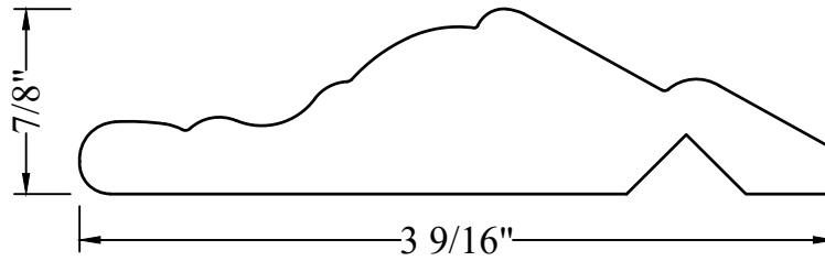
CC0018-00 CC0018-01 7/8" x 3 9/16"
